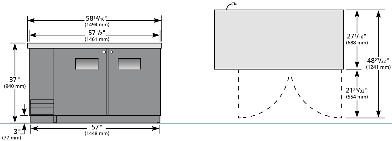
ELEVATION
