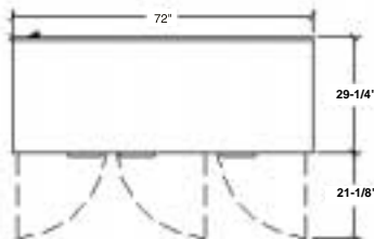
WTR72 Top
