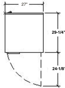
WTR27 Top
