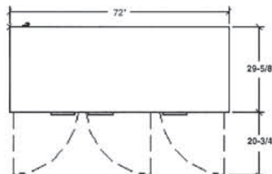
UCR72 Top
