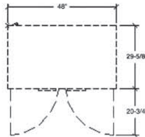
UCR48 Top
