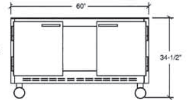
UCR60 Front
