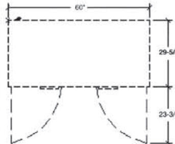
UCR60 Top
