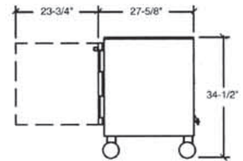
UCR-27SD End
