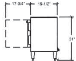
UCR-34 End
