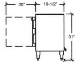
UCR/UCF-20 End
