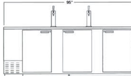
DD94 Front
